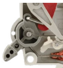
Автоматическая доводка рукоятки управления
